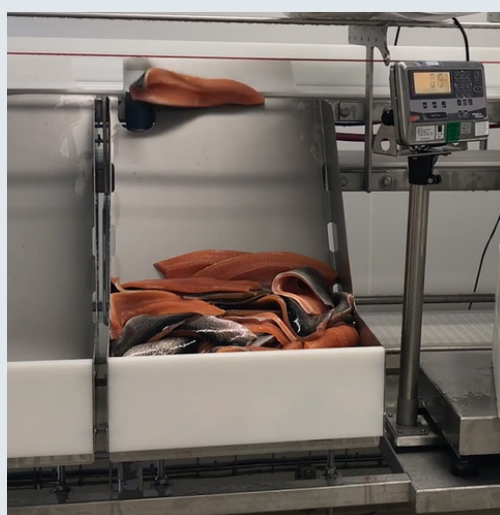
Calibreuse à truites mise en place chez l'un de nos clients
